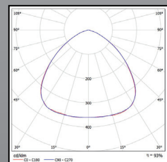
Fotometría diseñada para lograr una optima uniformidad lumínica
